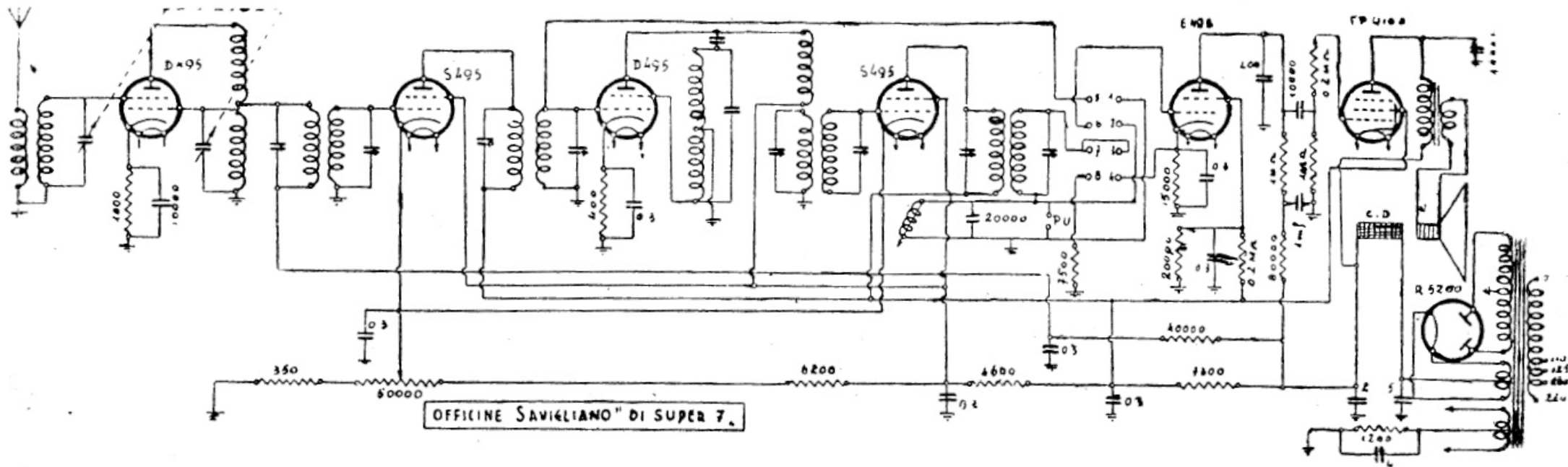
S. A. OFFICINE DI SAVIGLIANO — Modello « Di Super 7 » Produzione 1933.
